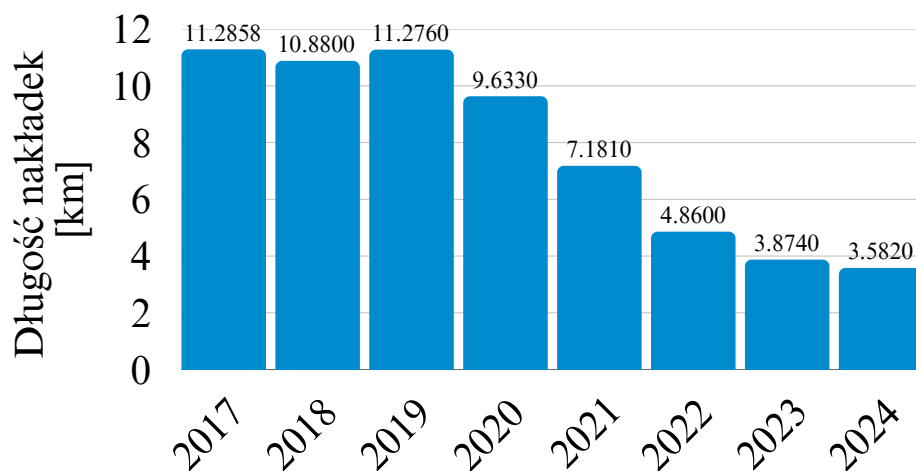
Rys. Długość wykonanych nakładek asfaltowych
