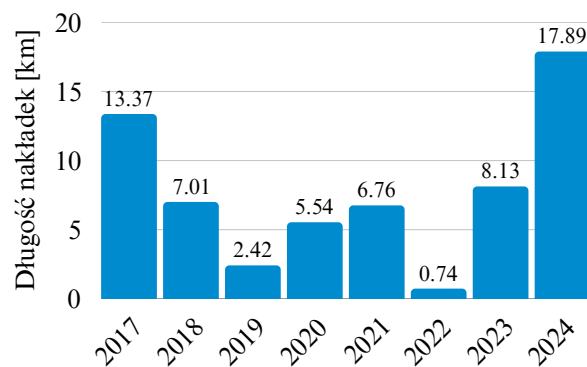
Rys. Wybudowane odcinki sieci kanalizacyjnej
